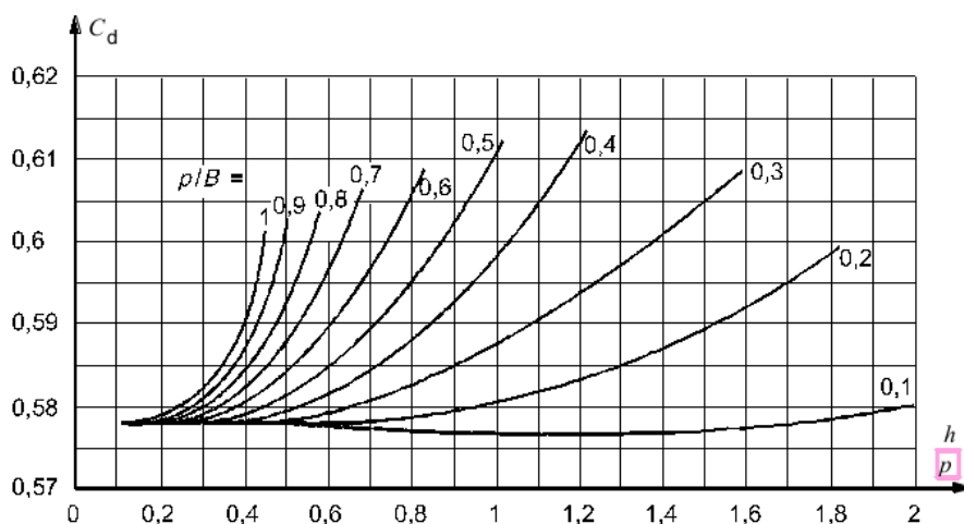
Hình B.4: Giá trị hệ số C_d theo tỷ số p/B với góc cửa tràn \alpha = 90^\circ
