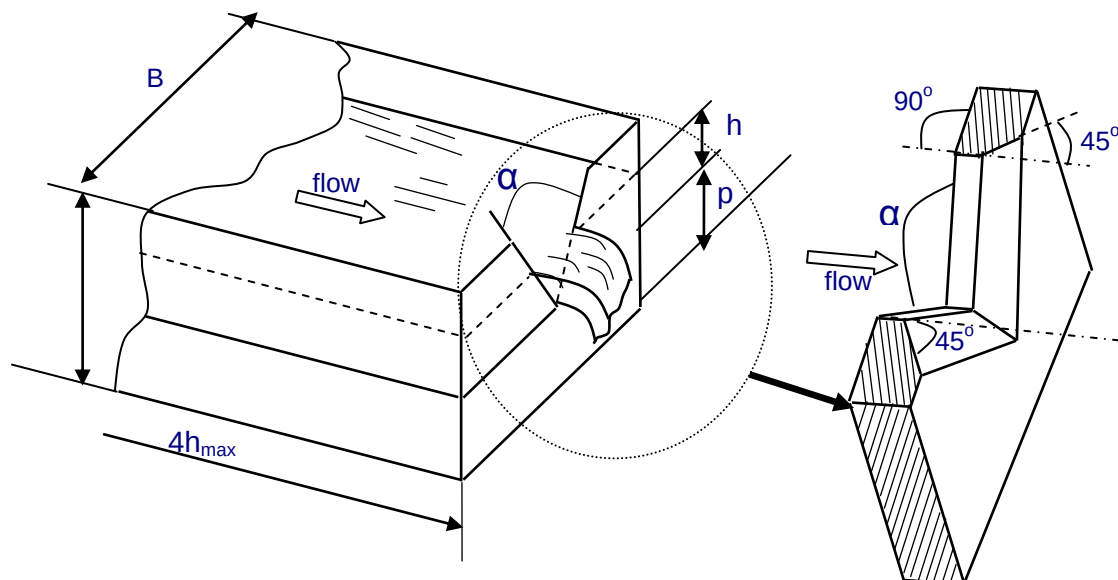
Hình A.2: Các kích thước và cấu tạo của đập tràn thành mỏng, cửa tràn hình tam giác
